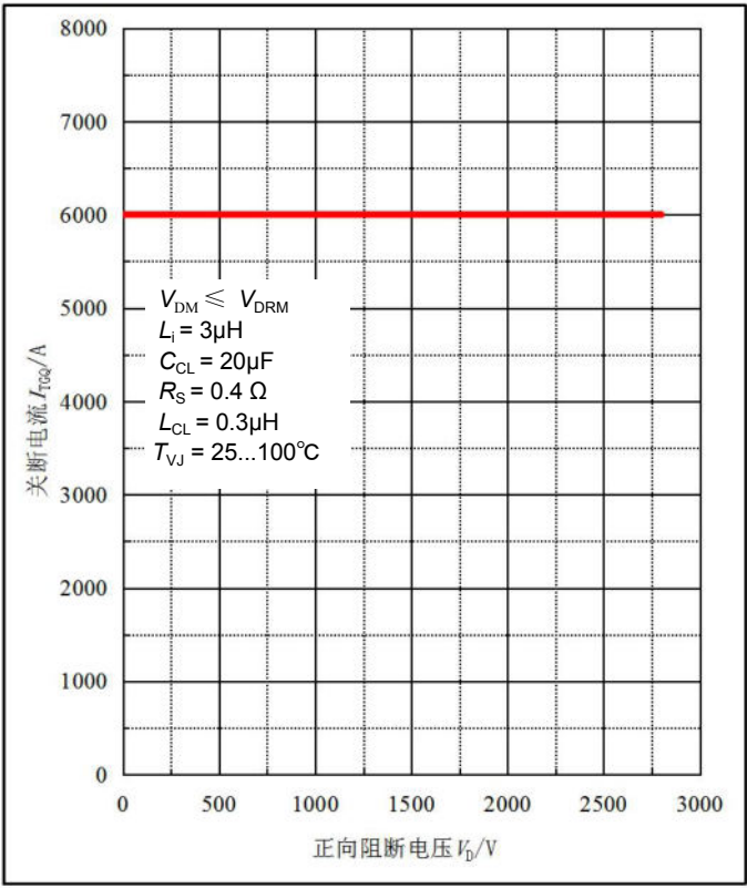
图4. 安全工作区
