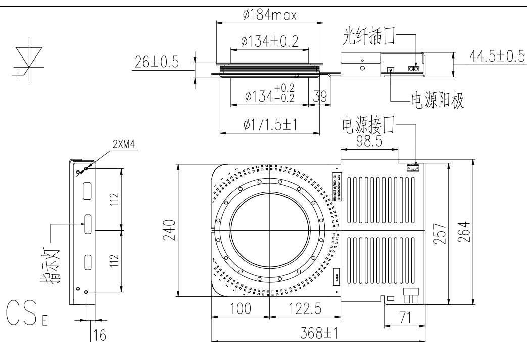
图8. IGCT外形图 (单位: mm)
